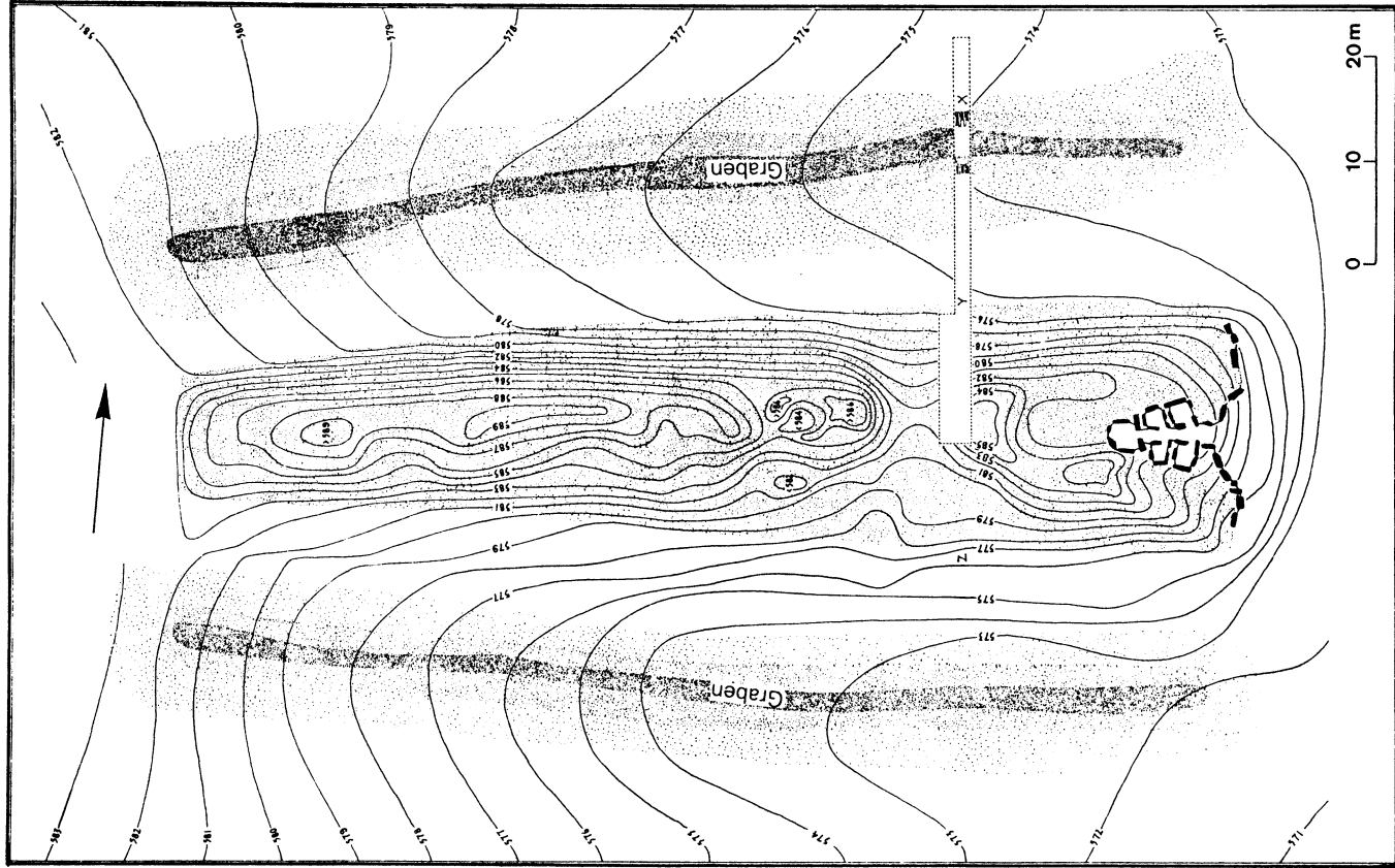
8 a West Kennet, Wiltshire, GB. Gesamtansicht.
