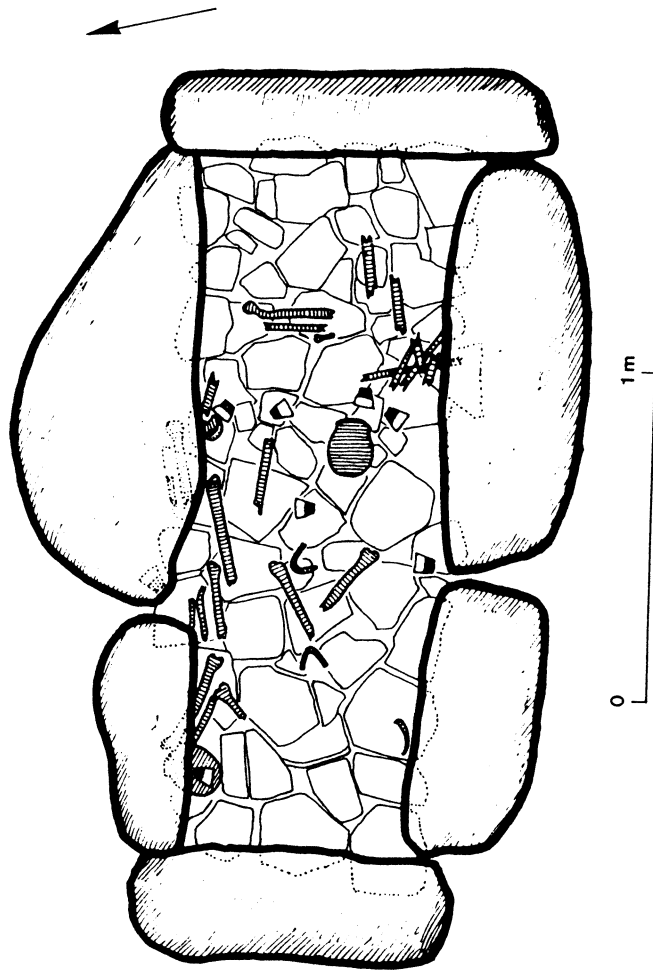
10a Everstorfer Forst, Kr. Grevesmühlen, Mecklenburg. Urdolmen bei Naschendorf.
